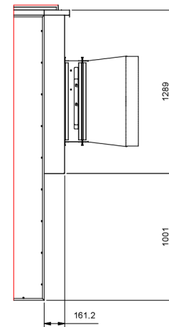
A ( 1 : 20 )
