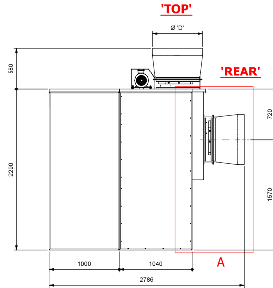
A ( 1 : 20 )
